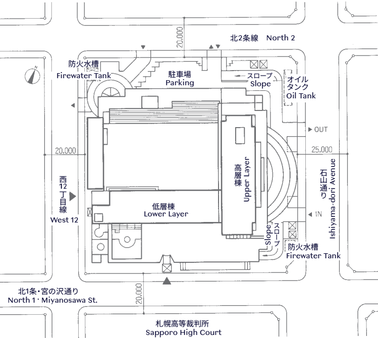
配置図 LOCATION
